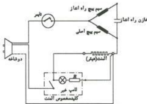
مدار الکتریکی لباسشویی نیمه اتوماتیک سطلی
