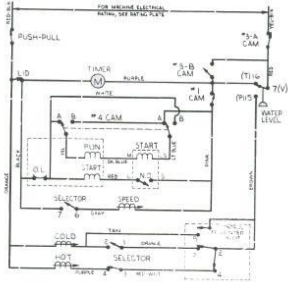
نقشه لباسشویی جنرال مدل: 96 D 560 (090)
