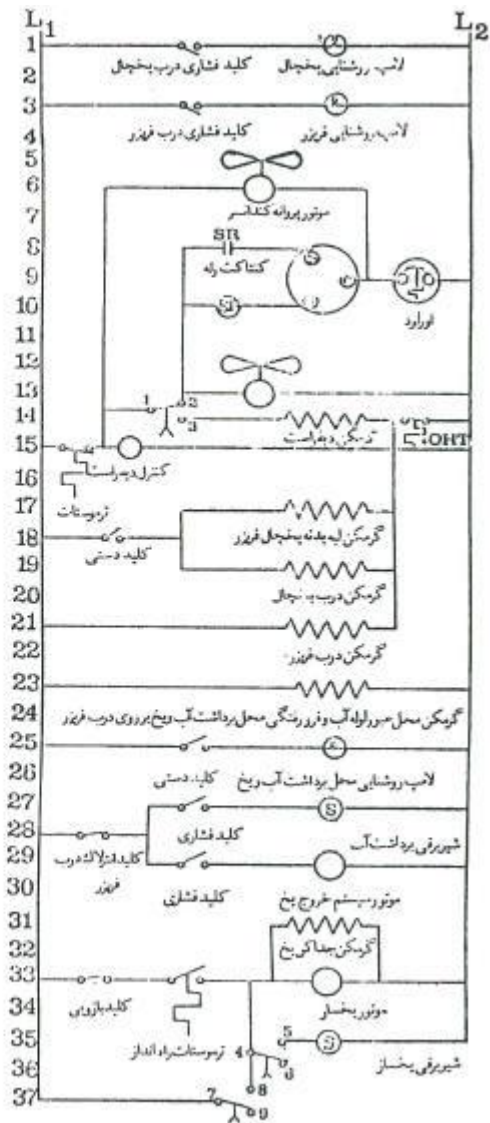
مدارهای الکتریکی یخچال فریزر خانگی مجهز به کنترل دیراست، آپریدن و یخساز
