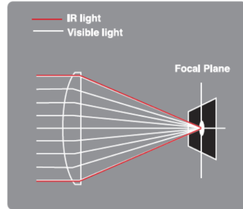
■ IR LENS
