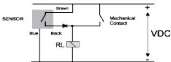
سه سیمه PNP موازی با کنتاکت مکانیکی
