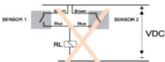
دو سیمه DC ( اتصال موازی مجاز نمی باشد. )
