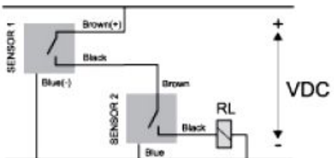
سه سیمه PNP
