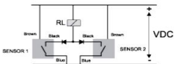
سه سیمه NPN
