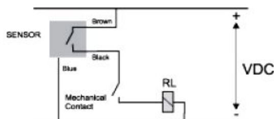
سه سیمه PNP سری با کنتاکت مکانیکی
