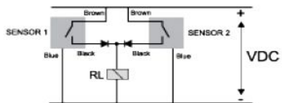
سه سیمه PNP
