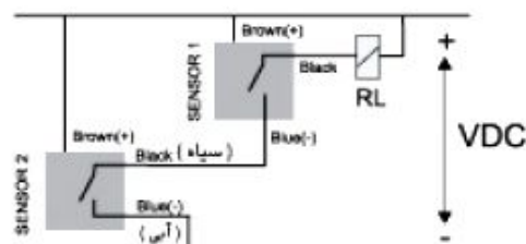
سه سیمه NPN
